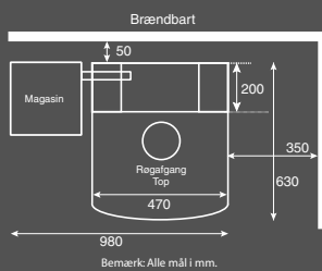
Måltegning - oppe
